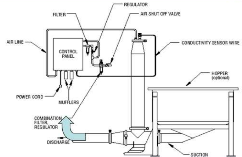
Sistema de Bombeo con Bomba VC
